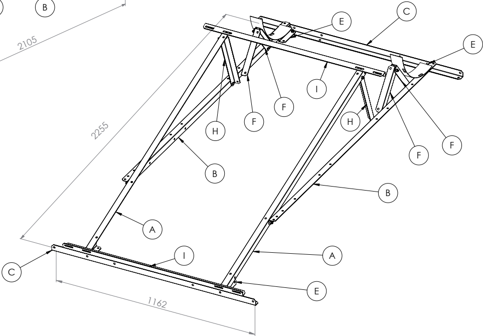
Cubierta inclinada Tilted roof
