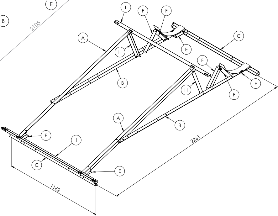
Cubierta inclinada Tilted roof
